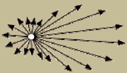
Mie Scattering
